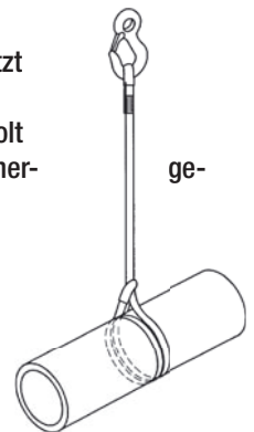
Bild D.2 - Doppelter Schnürgang
